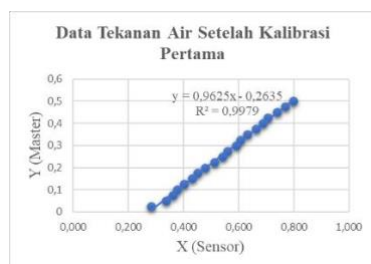
Gambar 18. Grafik Linearitas Sensor Pressure Transducer Kedua
