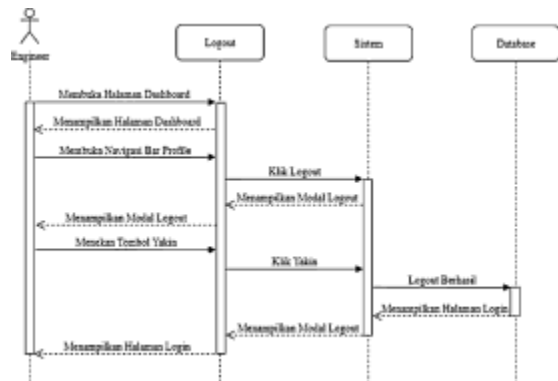
Gambar 22. Sequence Diagram Logout Engineer Setelah semua proses selesai, Engineer dapat keluar dari website dengan memilih menu Logout , yang akan mengarahkan kembali ke halaman Login .
