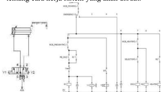
Gambar 4. Desain Sistem Kontrol Elektro Pneumatik
