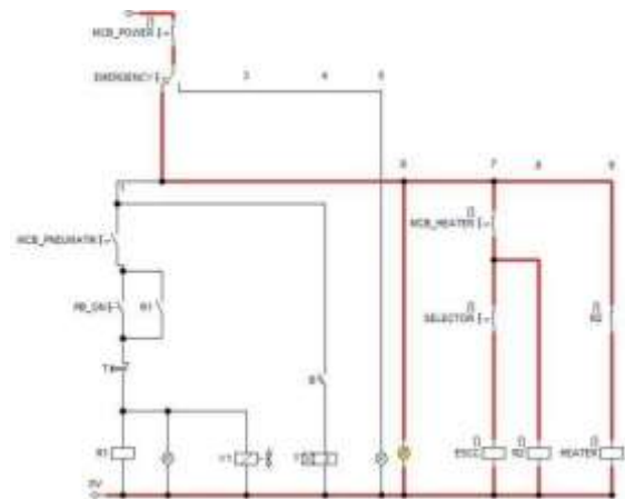
Gambar 10. Rangkaian Kondisi Heater On
