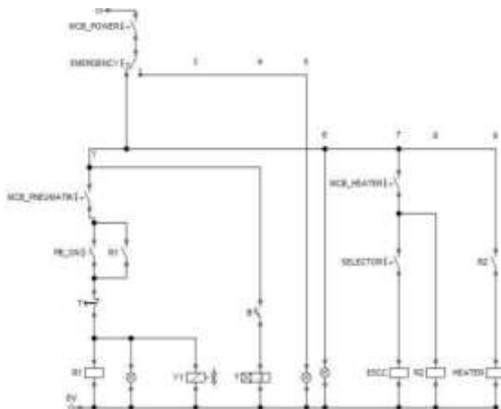
Gambar 9. Rangkaian Kondisi Heater Off
