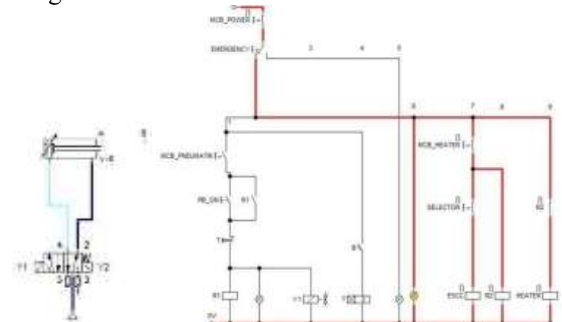
Gambar 11. Rangkaian Kondisi Pneumatik Off
