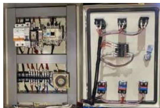
Gambar 7. Panel Kontrol Bagian Dalam
