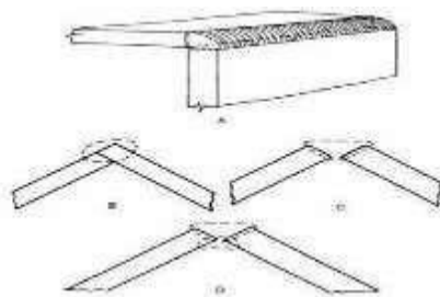
Gambar 6. Bentuk Sambungan Pengelasan Corner Joint ( Sumber : Simon Parkke, 2023)
