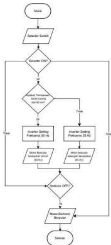
Gambar 12. Flow cara kerja alat
